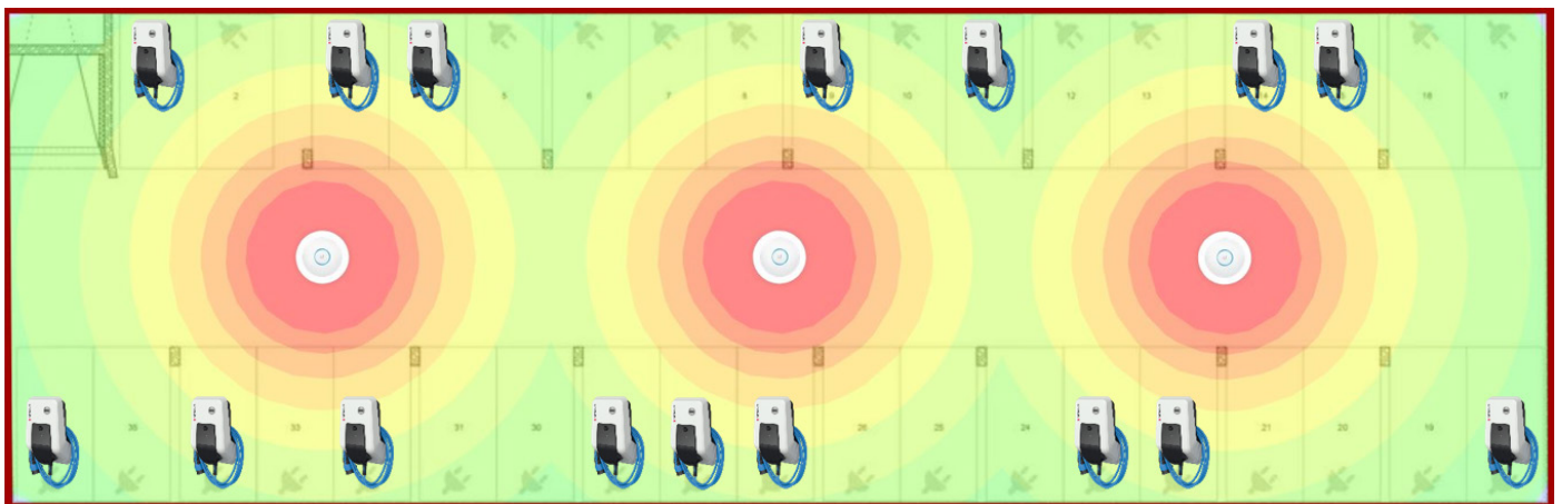
Planung und Simulation der WLAN Abdeckung und Vernetzung der Ladestationen
